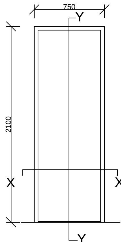
DOOR TYPE D2
