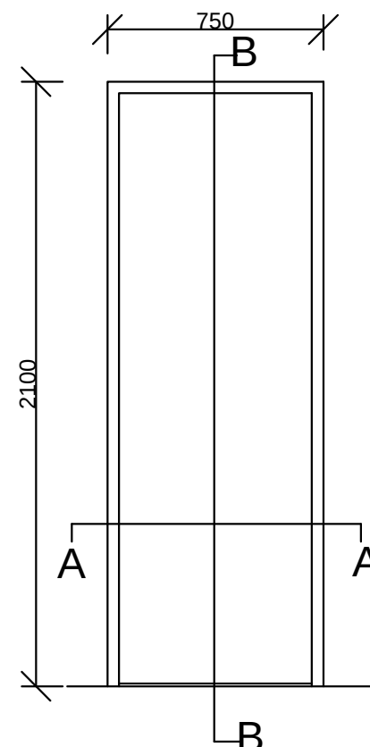
DOOR TYPE D3
