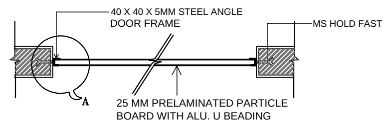
SECTION AT A-A N.T.S.
