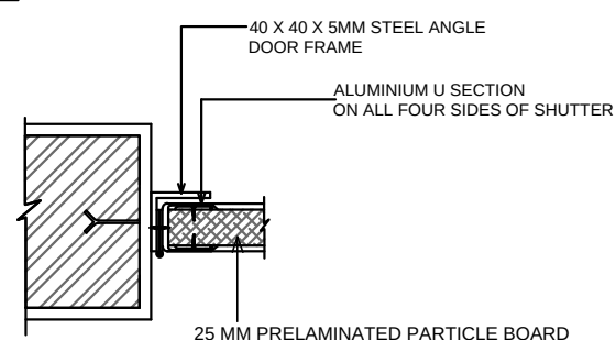
DETAIL AT A N.T.S.
