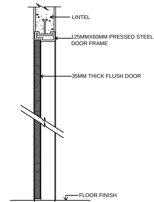
SECTION YY N.T.S.
