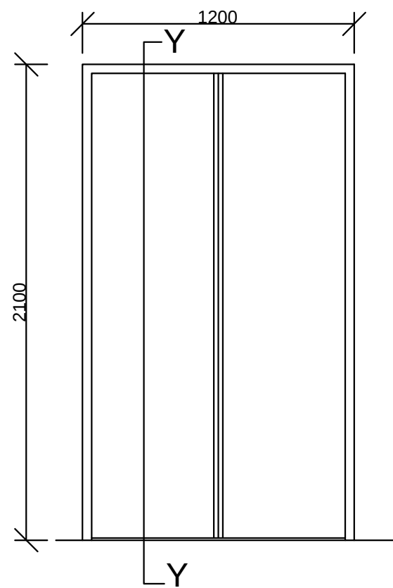
DOOR TYPE D
