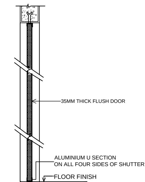
SECTION AT B-B N.T.S.
